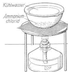
Abb. 3. Sublimation des Ammoniumchlorids.
